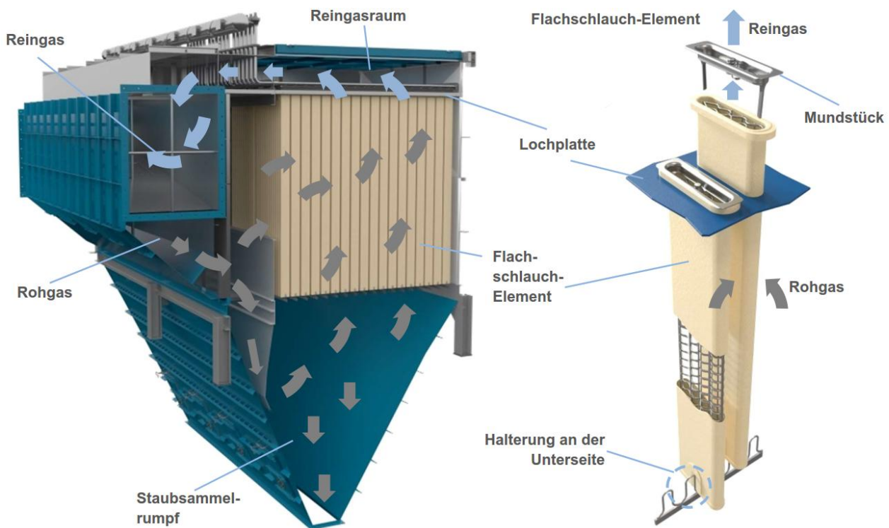
Abbildung 13 Beispielhafte Darstellung eines Gewebefilters (Quelle: LÜHR FILTER GmbH & Co KG)
