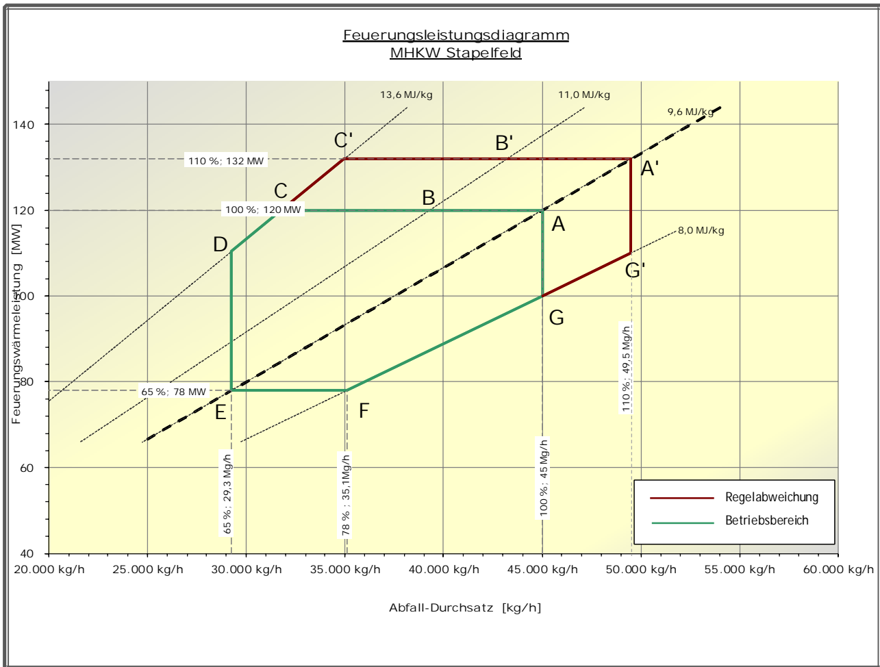
Abbildung 7 Feuerungs-Leistungs-Diagramm FLD
