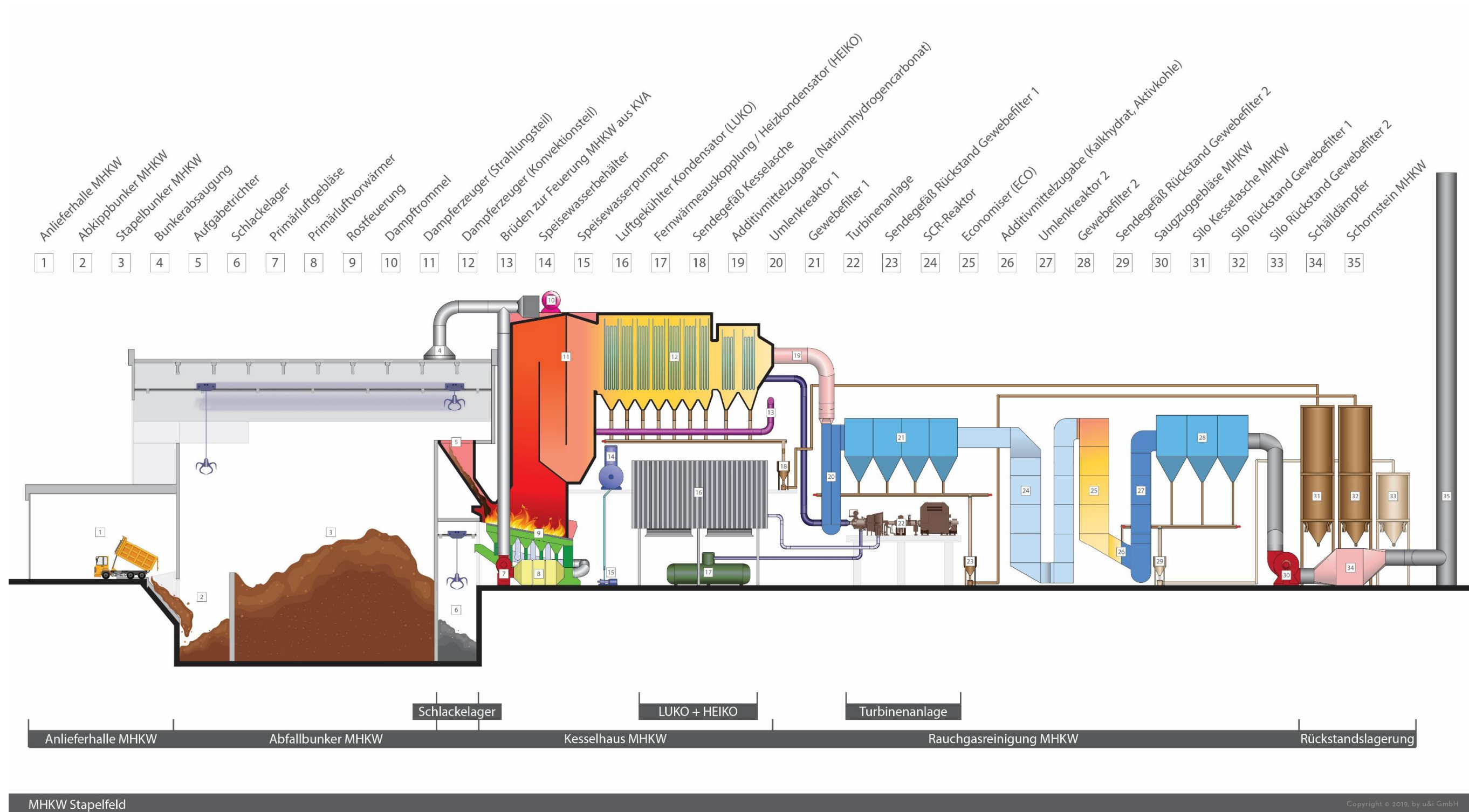
Abbildung 5 Darstellung der Verfahrenstechnik MHKW
